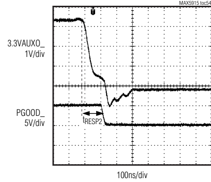
MAX5915A/MAX5916A 3.3VAUXO_SHORT CIRCUIT
